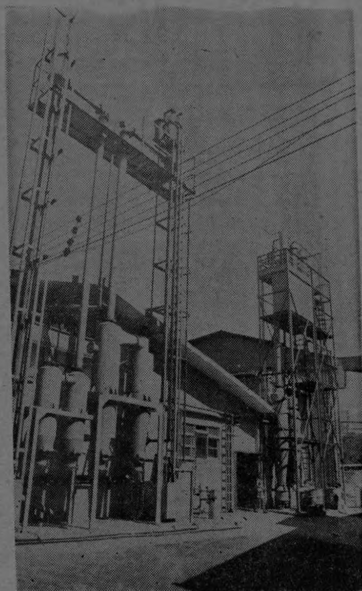
Vista parcial de TORRES DE VACIO, SECADO DEL JABON.
